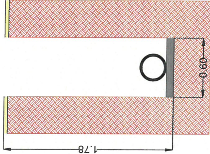
DETALLE DE INICIO DE EXCAVACION TRAMO 4
