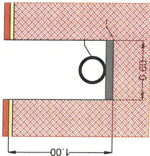
DETALLE DE TERMINO DE EXCAVACION TRAMO 4
