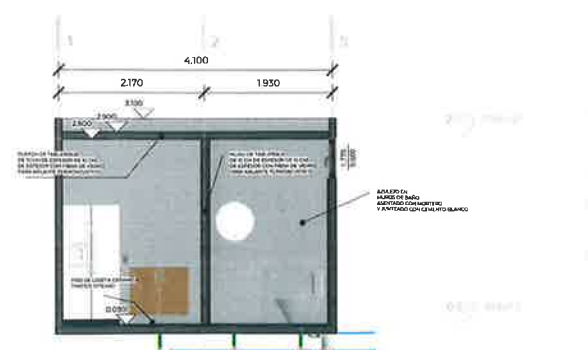
4 Sección 3 1:50
