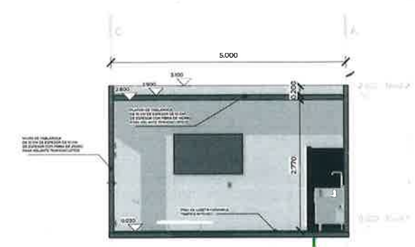
2 Sección 1 1:50
