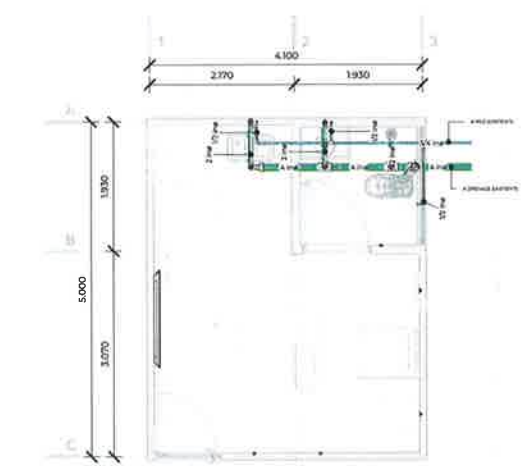
6 Hidrosanitario 1:50
