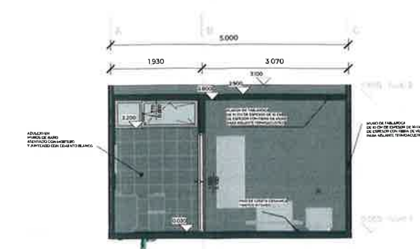
3 Sección 2 1:50
